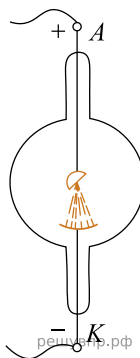
Рис. 1. Рентгеновская трубка
